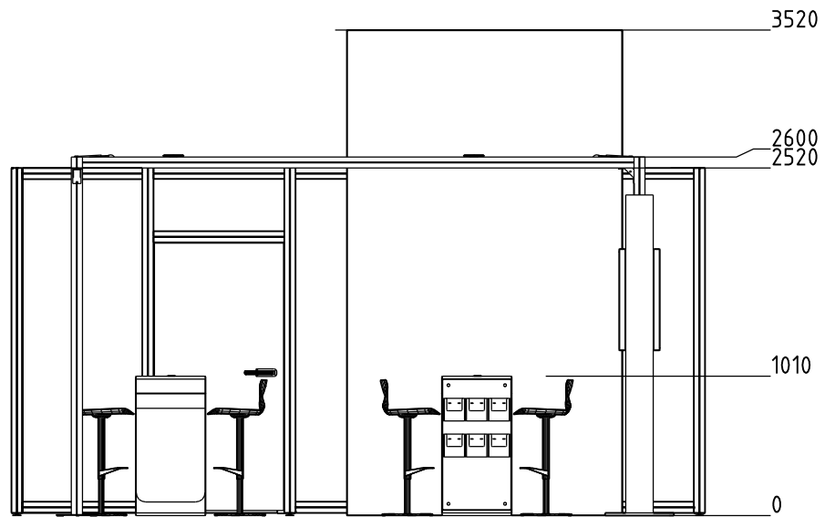
Höhenriss
