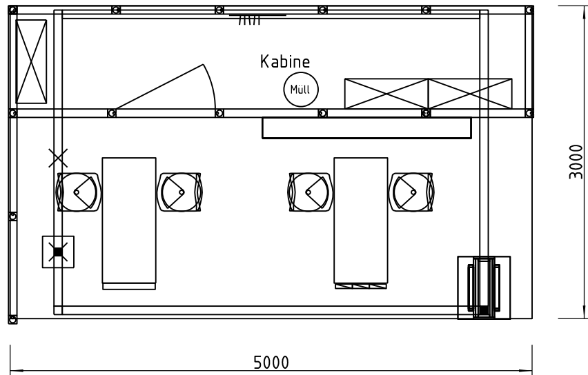
Grundriss
